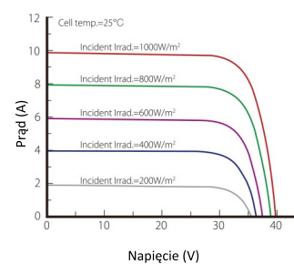
Wykres prąd-napięcie
