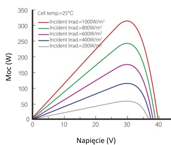
Wykres moc-napięcie
