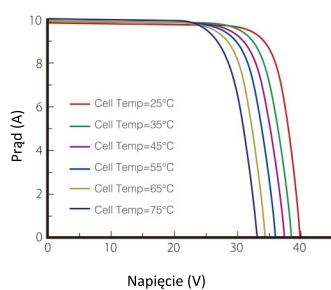
Wykres prąd-napięcie
